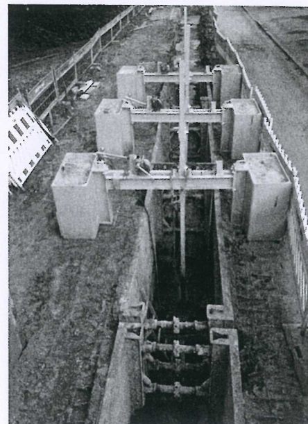
Abb. 6: Auftriebssicherung beim Einbringen von Flüssigboden
