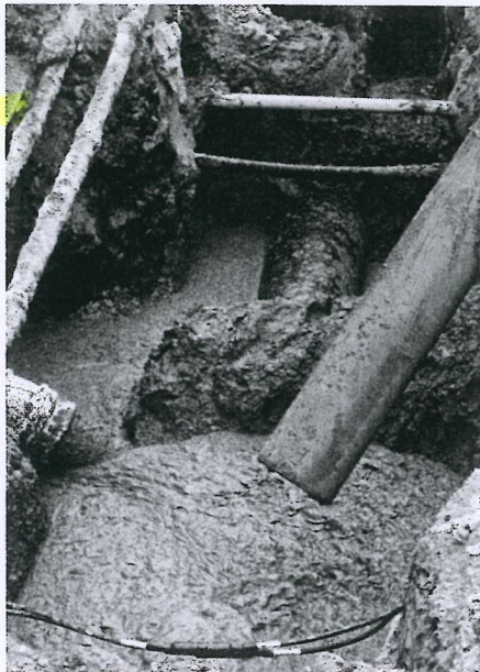
Abb. 5: Auflagerbänke und Auftriebssicherungen aus plastischem Material
